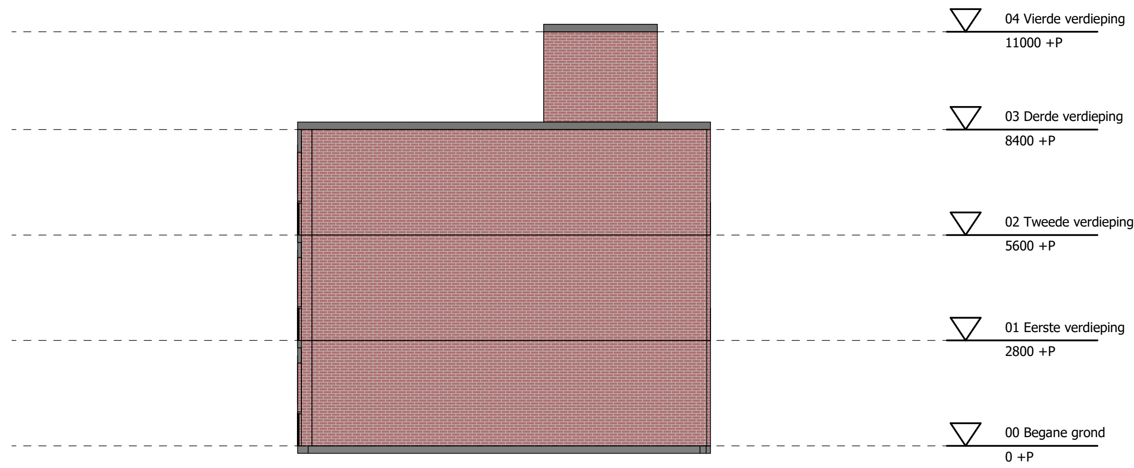
linkergevel
