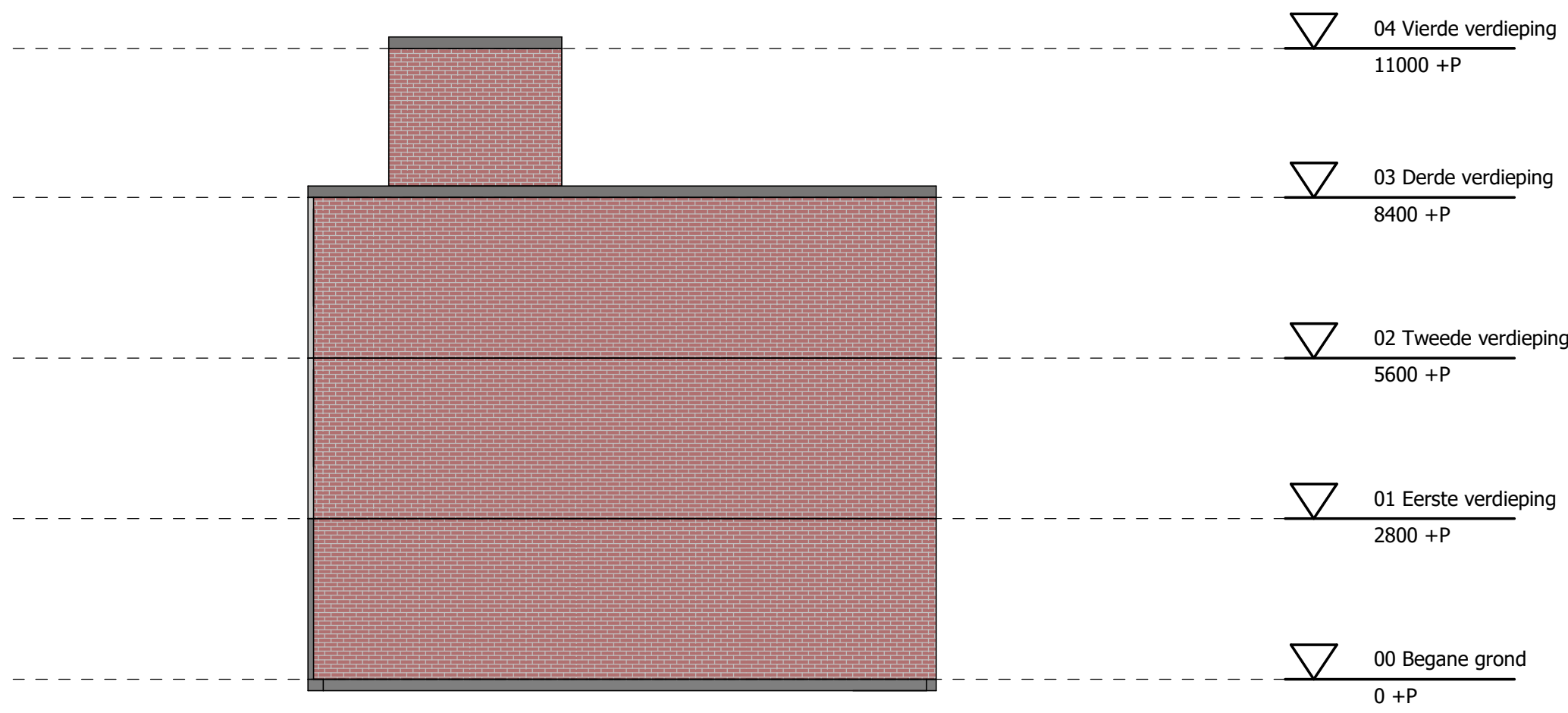
rechtergevel
