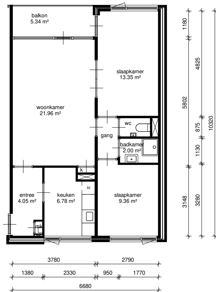
tweede verdieping
